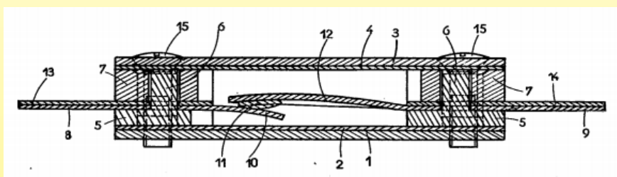
1961 биметаллический миниатюрный выключатель мгновенно действия для нагреваемых одеял, совместный патент Sté Augé et Cie и Imphy sa № FR1296066 (Франция)
