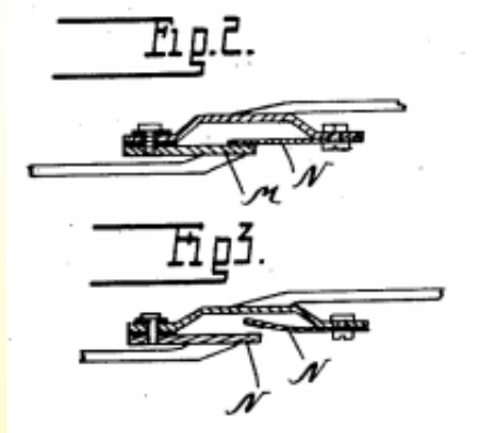
1912 Ограничитель из легкоплавкого сплава Хоффмана для нагревательного одеяла (патент США 1096916). Легкоплавкий сплав сваривает вместе лопасти M и N
