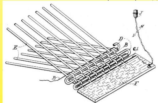
4 июня 1895 года, США. Патент №. 540398, Джон Эмори Мик из Денвера, для компании “Джонс Мэнүфэччуринг Сай” из Нью-Йорка, описал нагревательную ткань, нити основы которой (E) изготовлены из асбеста, а уточные пряжи (B) - из проводящего металла, со второй асбестовой прослойкой ткани (D). Два конца нагревательного элемента (F) не включают нагревательный провод.
