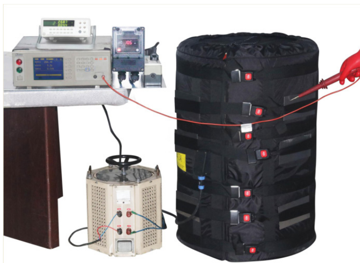
Измерительное оборудование для измерения полного тока утечки в горячем состоянии
