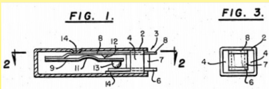
1963 Миниатюрный отщелкивающийся ограничитель Portage Electric (патент США 3443259). Его главной особенностью была регулировка заданного значения с помощью небольшого буртика в корпусе (№ 14), что было подхвачено большинством производителей.
