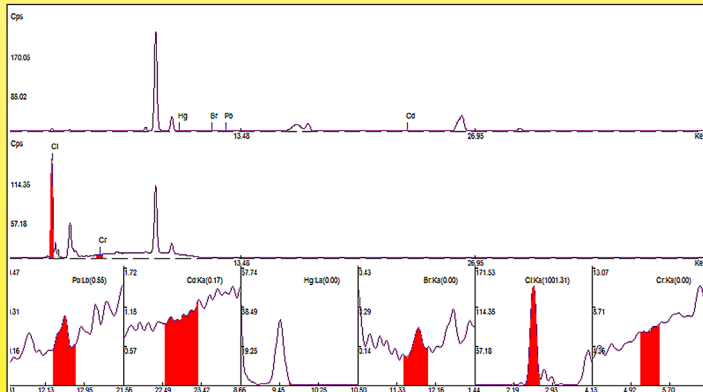
Спектрограмма Rohs изоляционного вспененного листа NBR-PVC (лаборатория Ul-timheat)
