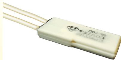
Водонепроницаемый биметаллический ограничитель Uchiya UP32 на нагревательном одеяле Gitem (коллекция Ultimheat).
