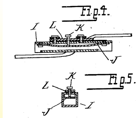
1912 Биметаллический термостат Хоффмана для согревающего одеяла (патент США 1096916). J представляет собой биметаллическую лопатку, заклепанную с обоих концов. Электрический контакт должен размыкаться между лопастью J, деформирующейся при повышении температуры, и установочным винтом K
