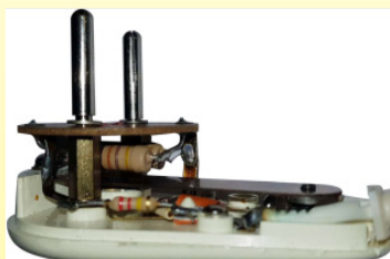
1972 г. Блок управления мощностью, изготовленный компанией Jidé в Лиможе под маркой Jidéstat. Самая успешная из всех систем. Очень маленькая по размеру, она регулируется и встроена в электрическую вилку. Это единственная модель с защелкивающимся магнитным контактом. Она не была превзойдена электромеханическими системами вплоть до нынешней эпохи. (Коллекция Ultimheat)
